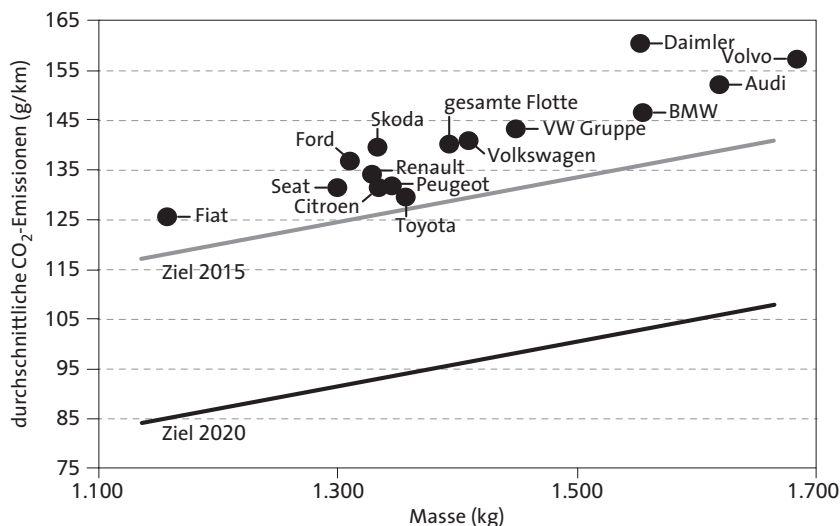
ABB. II.15 DURCHSCHNITTICHE CO 2 -EMISSIONEN DER HERSTELLER IM JAHR 2010 IM VERGLEICH ZU IHREN SPEZIFISCHEN GRENZWERTEN 2015 UND 2020
