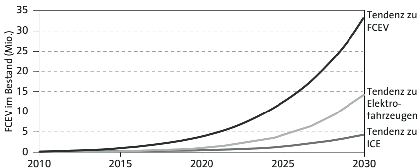
ABB. II.9 DREI MARKTHOCHLAUFSZENARIEN FÜR FCEV (WELTWEIT)
