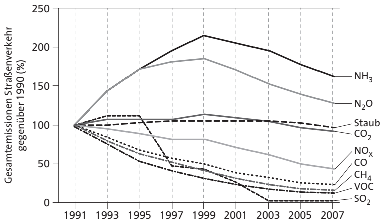
ABB. III.1 ENTWICKLUNG DER LUFTSCHADSTOFF- UND THG-EMISSIONEN DES STRASSENVERKEHRS
