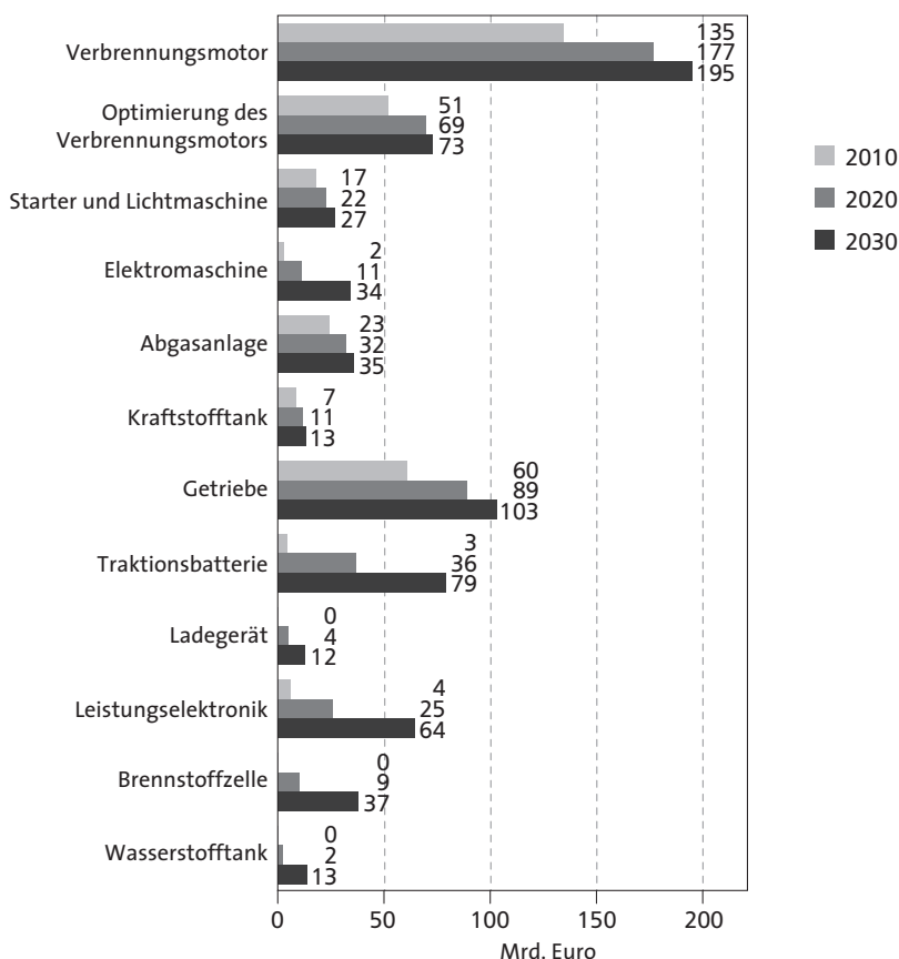
ABB. III.21 WERTSCHÖPFUNGSPOTENZIALE VON ZENTRALEN FAHRZEUGKOMPONENTEN
