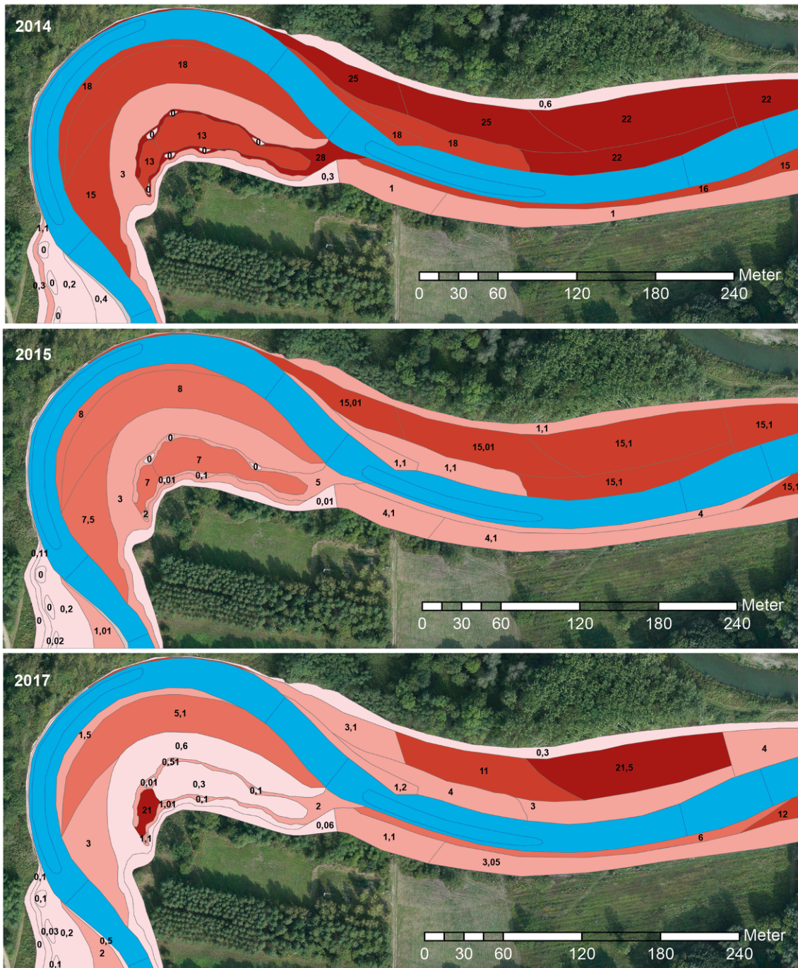
Abb. 6 Ausschnitt aus BA1 aus der flächendeckenden Kartierung Pflanzendichte der Schwarz-Pappel und Silber-Weide für die Jahre 2014, 2015 und 2017 (Datenquelle Aigner et al. 2014; Kreuzberger 2017; Egger und Mayer 2018; verändert aus: Mayer 2018)
