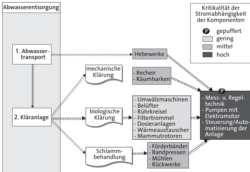
ABB. 18 ÜBERSICHT DER TECHNISCHEN ELEMENTE IN DER ABWASSERENTSORGUNG UND DER STROMABHÄNGIGKEIT
